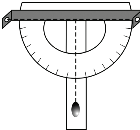
Рис. 3.3. Найпростіший висотомір
