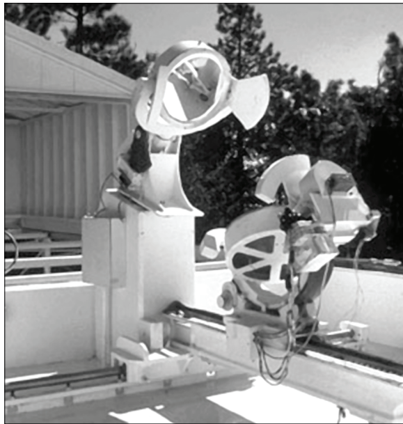
Рис. 9.8. Целостат сонячного телескопа
