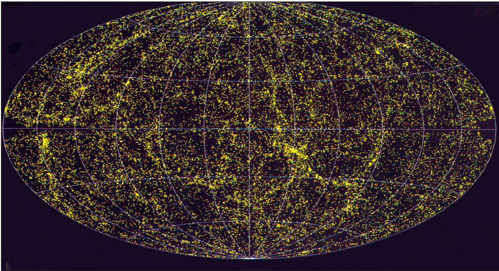
Рис. 20.16. Комірчастий розподіл галактик у просторі
