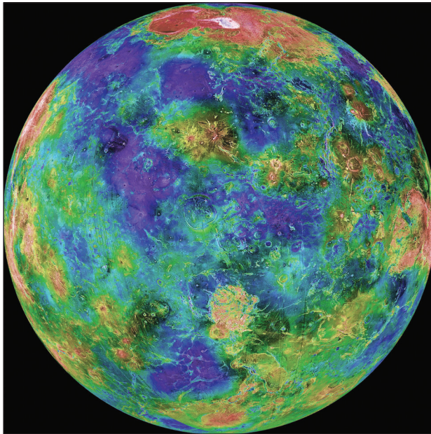
Рис. 12.4. Радіолокаційна карта поверхні Венери
