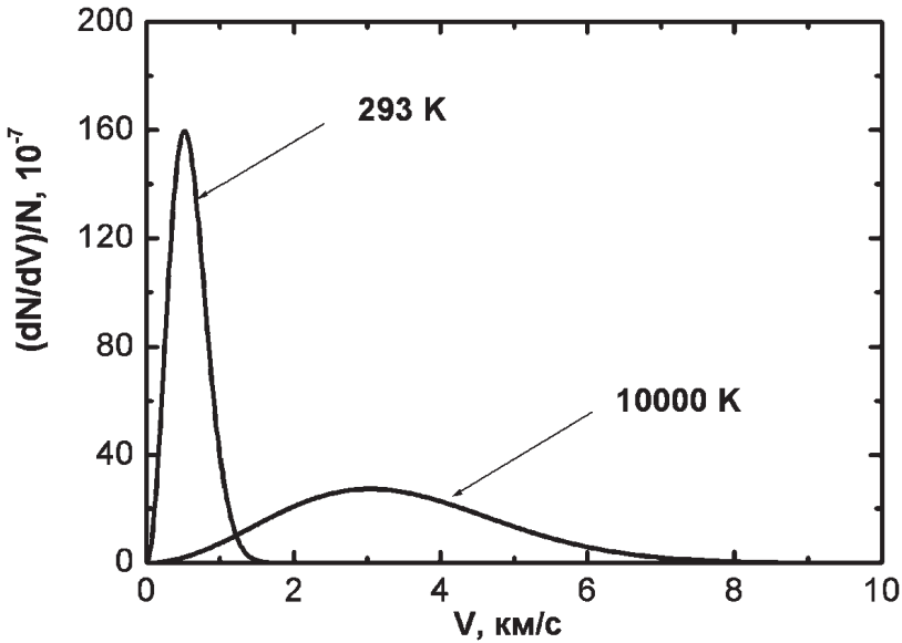
Рис. 8.5. Розподіл атомів фтору за швидкостями при температурах 293 К і 10 000 К; по осі абсцис відкладено швидкості частинок газу, по осі ординат — кількість частинок, що мають певну швидкість при заданій температурі, нормовану на повну кількість частинок фтору
