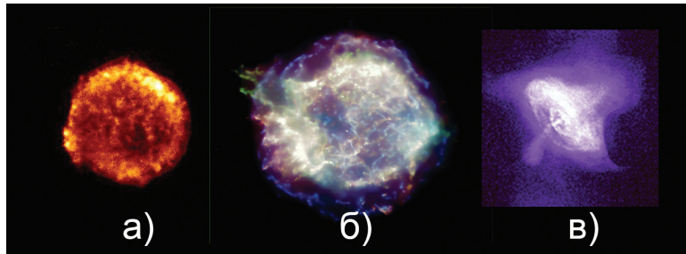
Рис. 17.4. Залишки спалахів Наднових у рентгенівських променях: а) — залишок Наднової 1572 р. (вперше поміченої В. Шулером і описаної Тихо Браге) — тип Ia, б) — залишок Наднової II типу Кассіопея А (вперше її спостерігав Дж. Флемстід у 1680 р.), в) — залишок Наднової II типу 1054 року — Крабоподібна туманність
