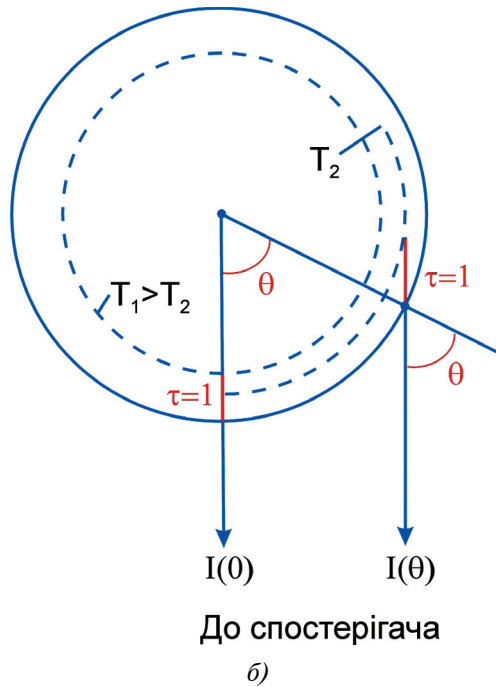
Рис. 11.3. Потемніння диска Сонця до його краю: а — фотографія Сонця, б — схематичне пояснення потемніння видимого диска до його краю
