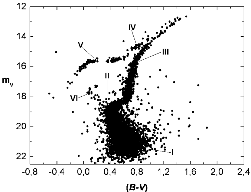
Рис. 19.3. Діаграма колір — зоряна величина для кулястого зоряного скупчення M\ 3 (NGC 5272) з сузір'я Гончих Псів. I — головна послідовність, II — точка повороту від головної послідовності, III — вітка червоних гігантів, IV — асимптотична вітка гігантів, V — горизонтальна вітка з провалом Шварцшильда, VI — блакитні бродяги
