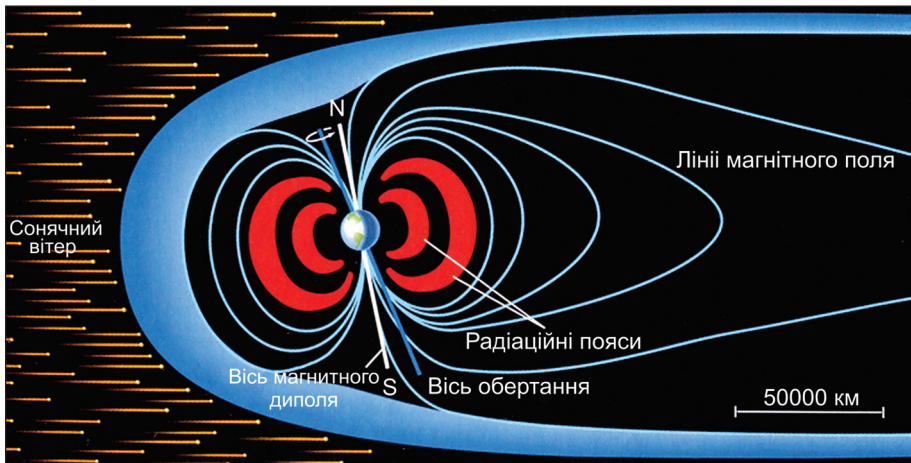
Рис. 12.6. Магнітосфера Землі
