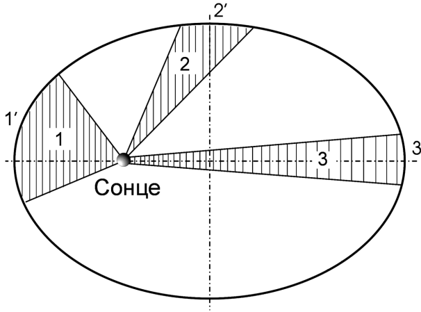
Рис. 4.12. Ілюстрація до другого закону Кеплера: площі 1, 2 і 3 — рівновеликі, це означає, що по дузі 1' планета рухається з більшою швидкістю, ніж по дугах 2' і 3'
