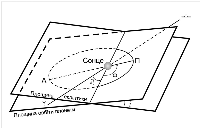
Рис. 4.13. Елементи планетної орбіти
