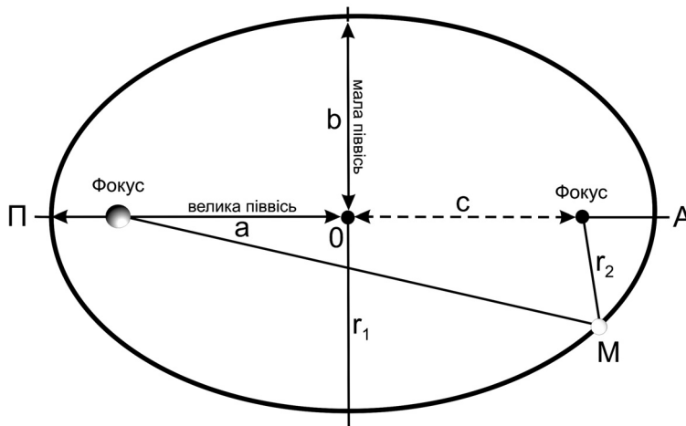
Рис. 4.11. Еліпс як орбіта планети; сума радіусів-векторів r_1 і r_2 будь-якої точки еліпса M дорівнює його великій осі
