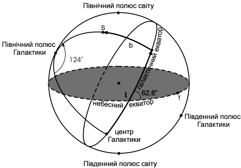
Рис. 19.1. Галактична система координат, S — зоря з координатами l і b
