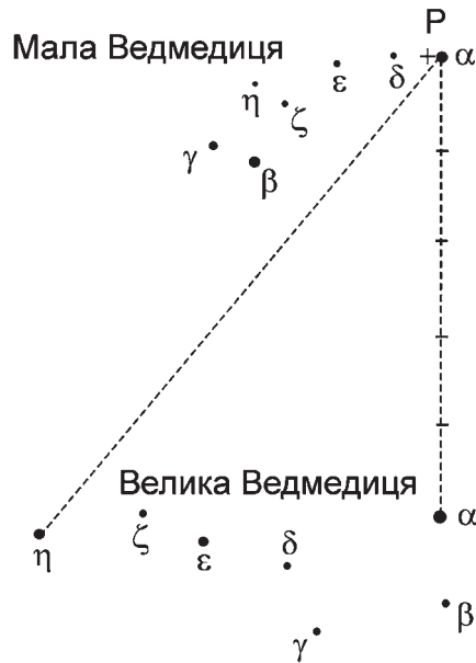
Рис. 1.4. Положення північного полюса світу серед зір
