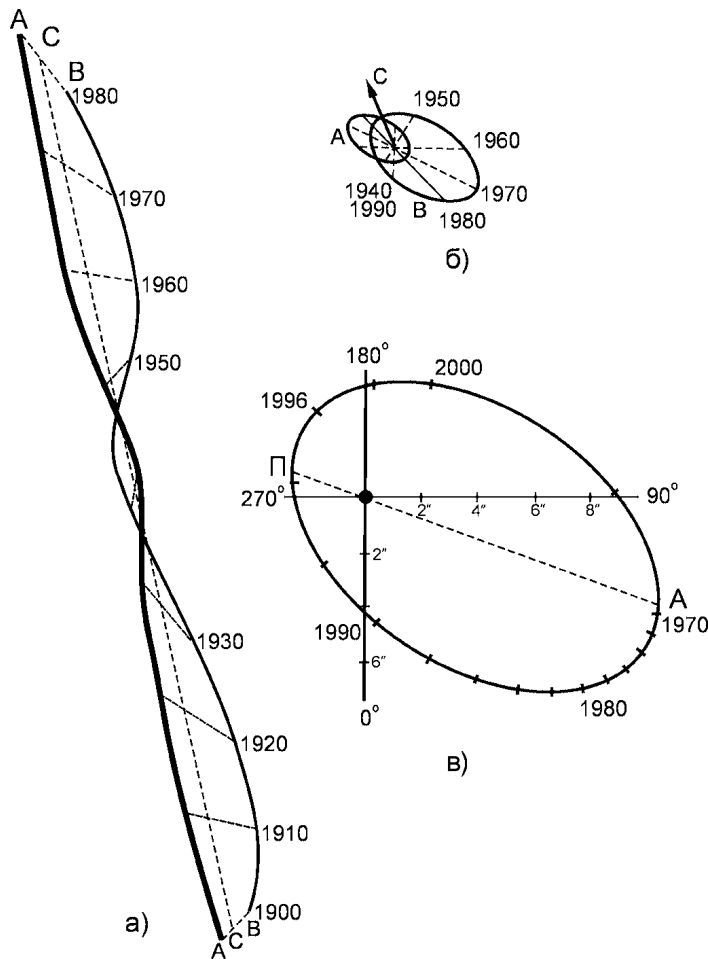
Рис. 15.10. Рух Сіріуса та його супутника: а) — видимий рух Сіріуса на загальному фоні далеких зір (жирна лінія), його супутника (тонка лінія) і їхнього центра мас (штрих) від 1870 року до 1980 року; б) — видимі орбіти обох зір, що рухаються навколо спільного центра мас; в) — орбіта супутника, який рухається відносно головної зорі
