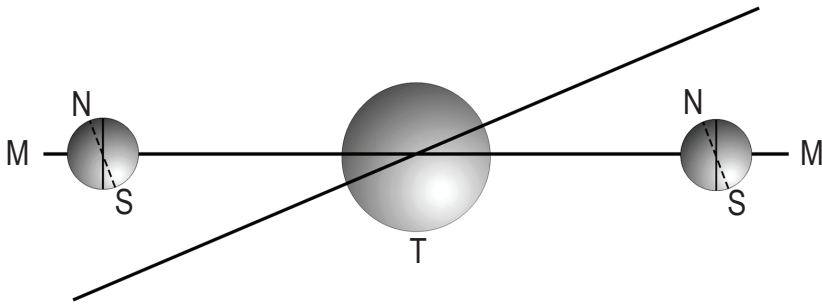
Рис. 5.4. Лібрація Місяця по широті
