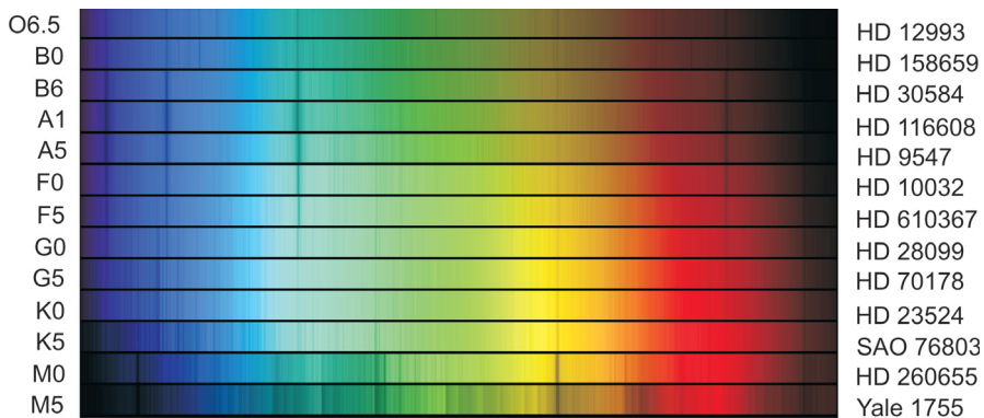
Рис. 14.3. Спектри зір різних спектральних класів; зліва вказаний спектральний клас, справа — номер зорі за каталогом
