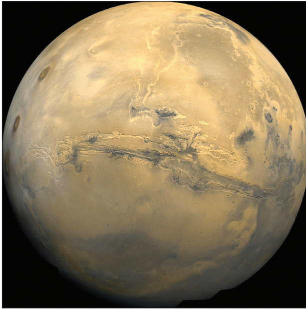
Рис. 12.9. Фото Марса
