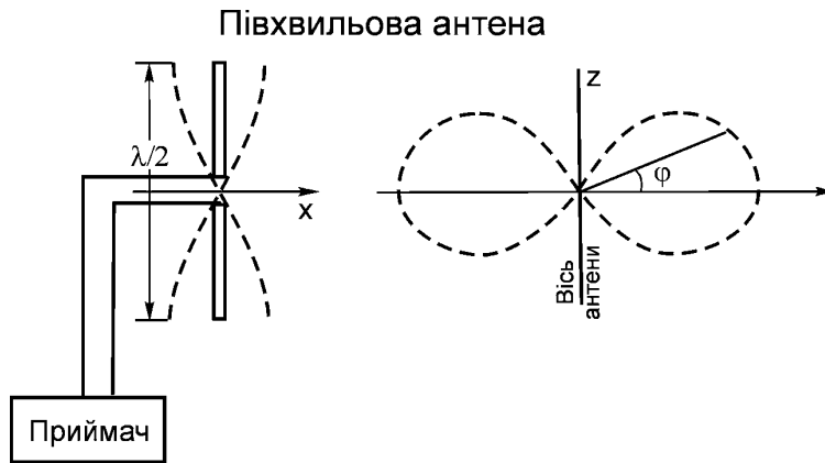
Рис. 9.9. Півхвильовий диполь і його діаграма направленості
