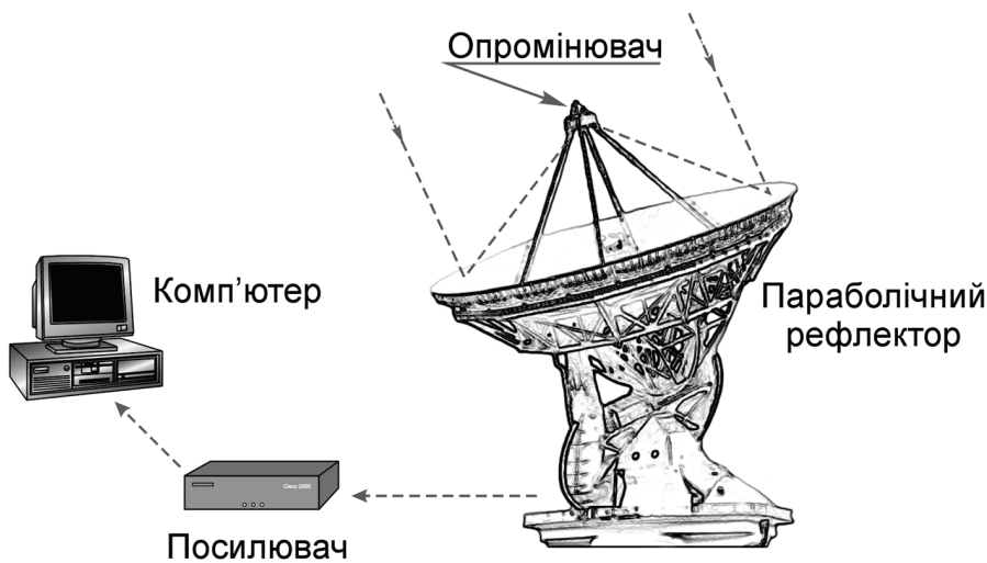
Рис. 9.10. Параболічна антена
