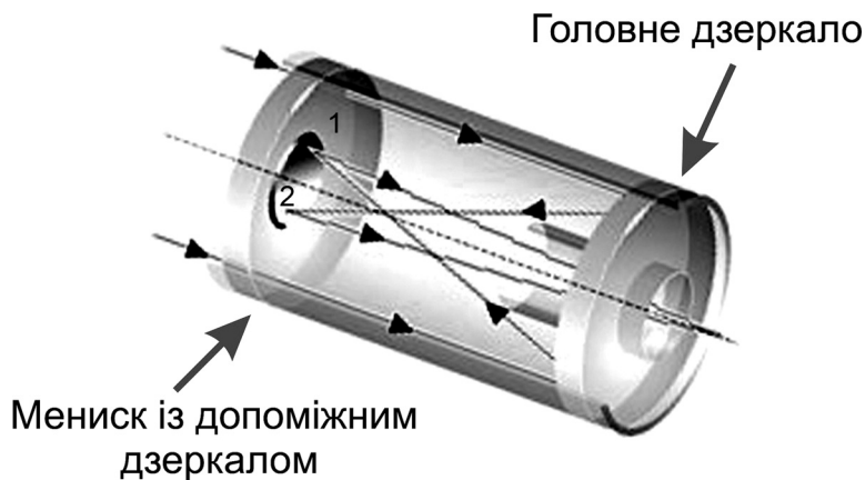
Рис. 9.5. Схема меніскової системи Максутава: 1 — сферичний мениск; 2 — опукле дзеркало
