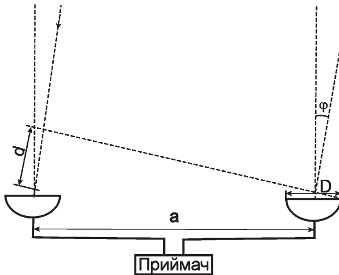
Рис. 9.11. Схема двохантного радіоінтерферометра
