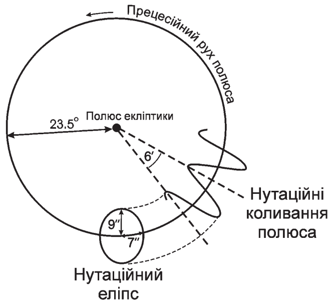
Рис. 1.21. Рух полюса світу внаслідок прецесії і нутації
