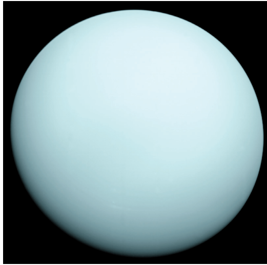
Рис. 12.18. Уран
