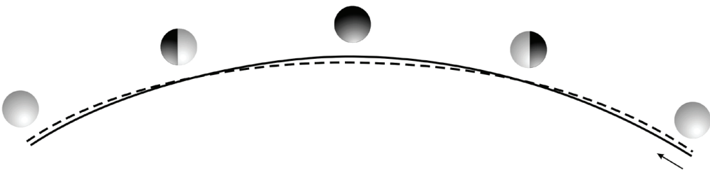
Рис. 5.3. Траєкторія Землі (суцільна лінія) і Місяця (пунктир) відносно Сонця. Вказані фази Місяця
