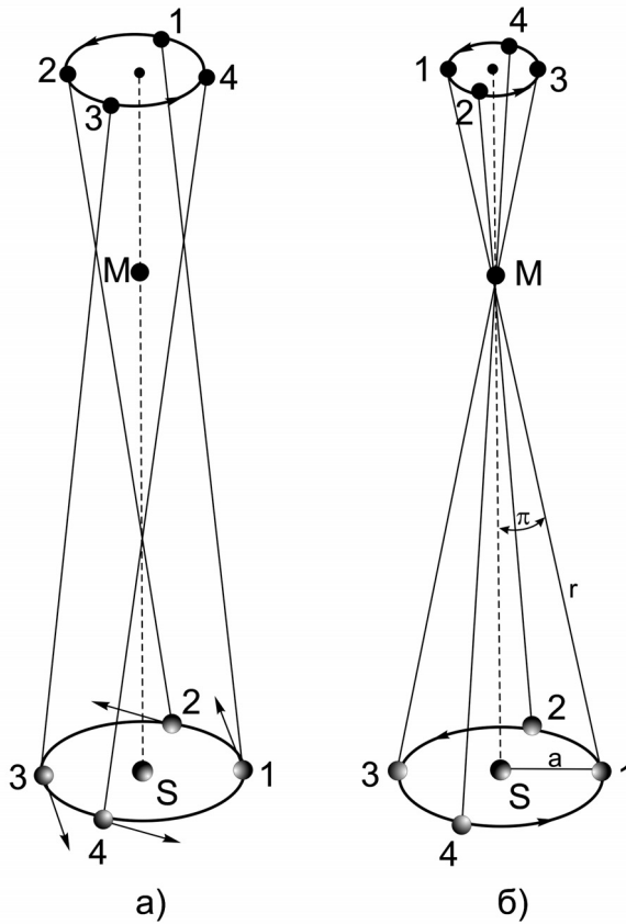
Рис. 4.18. Абераційне (а) і паралактичне (б) зміщення зорі протягом року; S — положення Сонця
