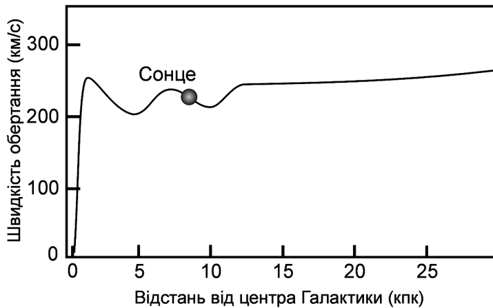
Рис. 19.8. Розподіл швидкостей обертання зір і газу у диску Галактики
