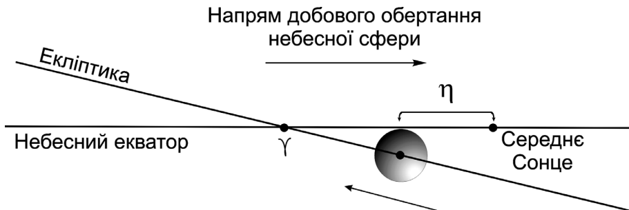
Рис. 2.6. Положення справжнього Сонця і середнього екваторіального Сонця в середині березня
