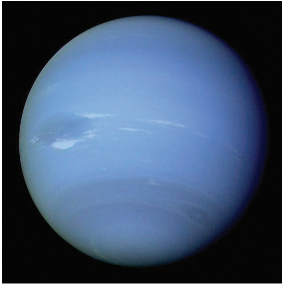
Рис. 12.19. Нептун
