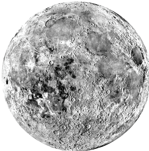
Рис. 12.7. Місяць
