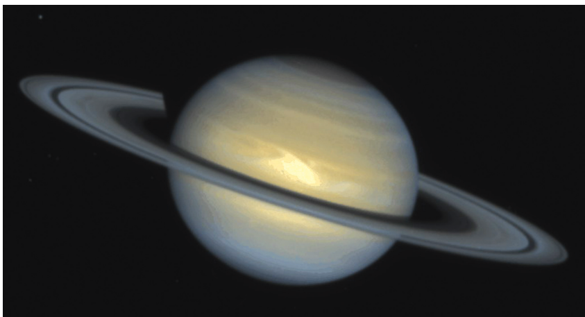
Рис. 12.16. Сатурн
