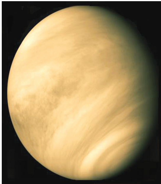
Рис. 12.3. Венера
