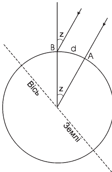
Рис. 3.4. Визначення радіуса Землі за допомогою вимірювання зенітної відстані світила з двох пунктів
