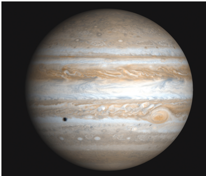
Рис. 12.14. Юпітер
