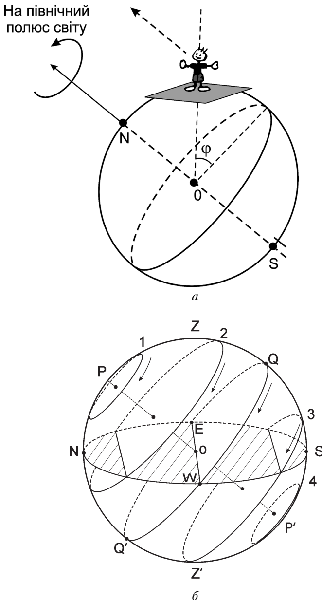
Рис. 1.12. Спостерігач середньої географічної широти ( a ) і його небесна сфера ( b )
