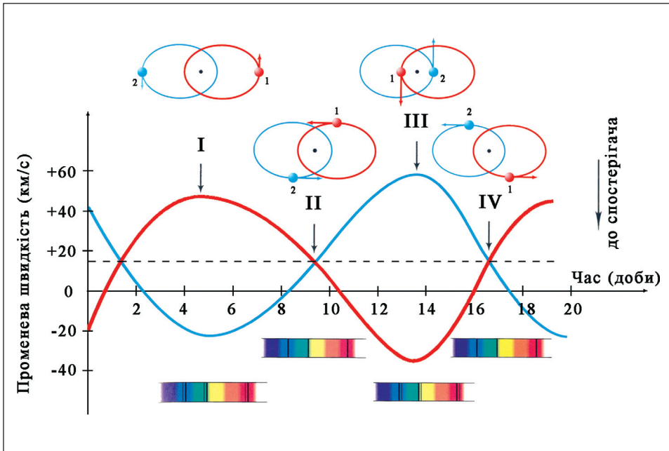
Рис. 15.5. Схема зміни променевої швидкостей у системі спектрально-подвійної зорі і періодичного зміщення спектральних ліній (внизу). Обидві зорі тут мають однакові маси, а отже амплітуда коливань променевої швидкості буде однаковою. Римські числа позначають відповідність спектрів положенню зір на їх орбітах. Горизонтальна штрихова лінія позначає променево швидкість руху центра мас системи відносно спостерігача
