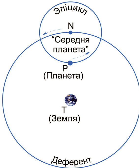
Рис. 4.3. Епіцикл і деферент у системі світу Птолемея
