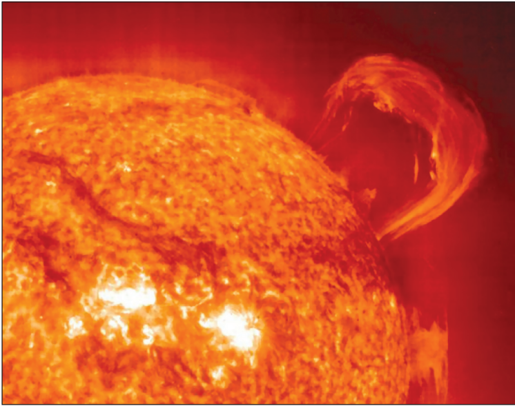
Рис. 11.9. Сонячний протуберанець
