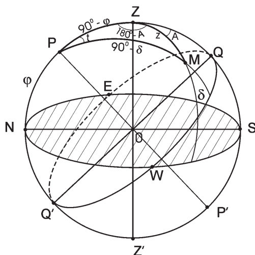
Рис. 1.17. Паралактичний трикутник
