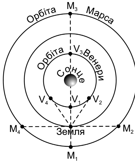
Рис. 4.2. Конфігурації планет
