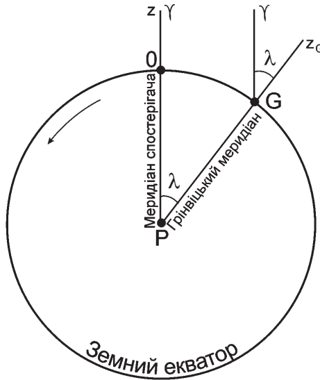
Рис. 1.5. Визначення зв'язку між місцевим s і грінвіцьким s_0 зоряним часом: якщо для спостерігача O точка весняного рівнодення у даний момент перебуває у верхній кульмінації, то для спостерігача G її верхня кульмінація відбудеться через проміжок часу, за який Земля повернеться на кут \lambda
