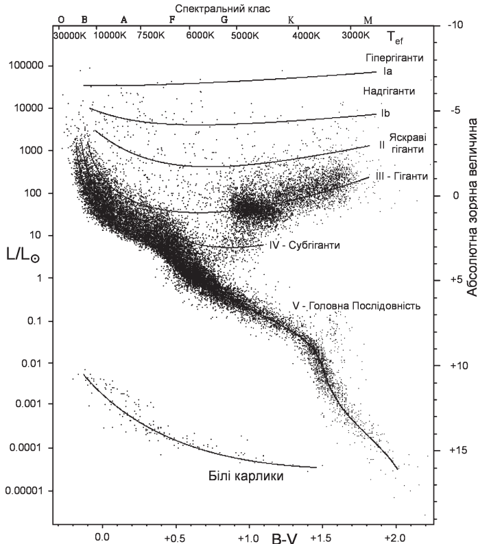
Рис. 14.4. Діаграма спектральний клас — світність
