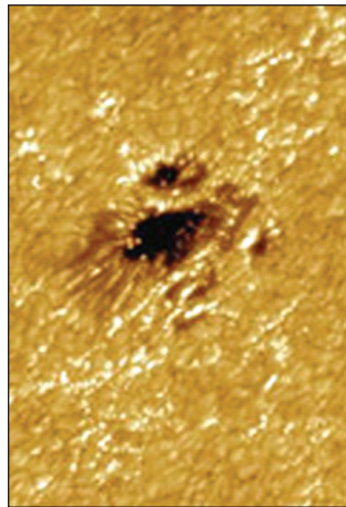
Рис. 11.8. Світлі факели навколо сонячної плями
