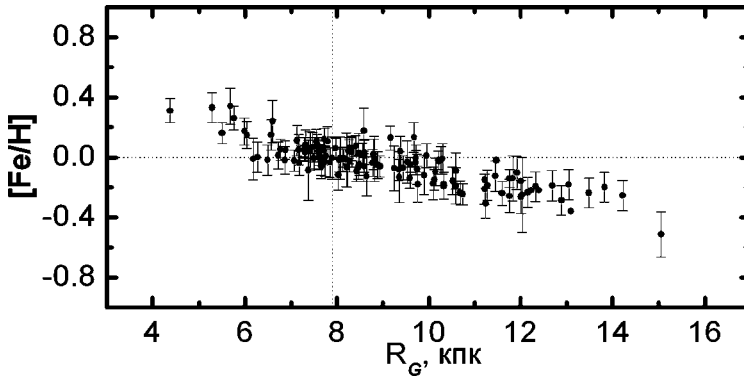
Рис. 19.12. Розподіл відносного вмісту заліза в атмосферах зір у диску Галактики за даними про галактичні цефеїди; положення Сонця вказано перетином двох крапкових ліній
