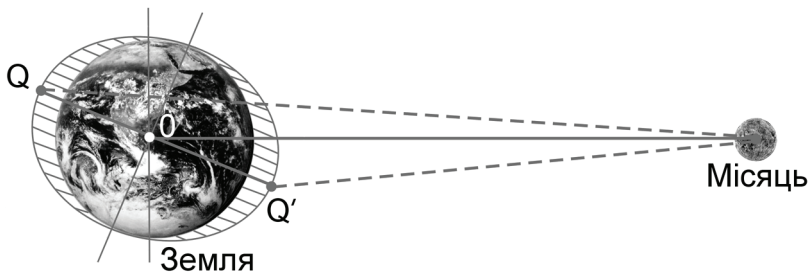
Рис. 6.7. Пояснення прецесії
