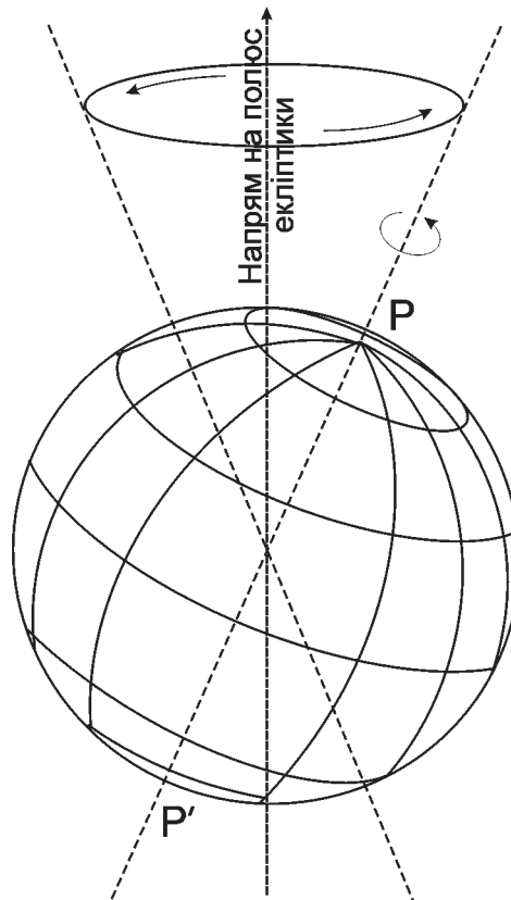
Рис. 1.19. Явище прецесії
