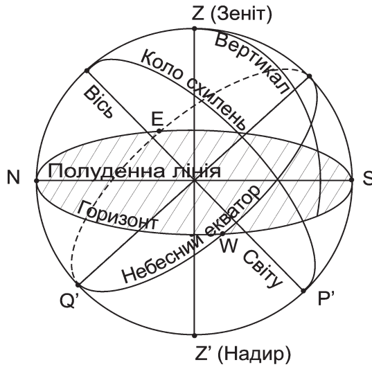
Рис. 1.3. Точки і лінії небесної сфери
