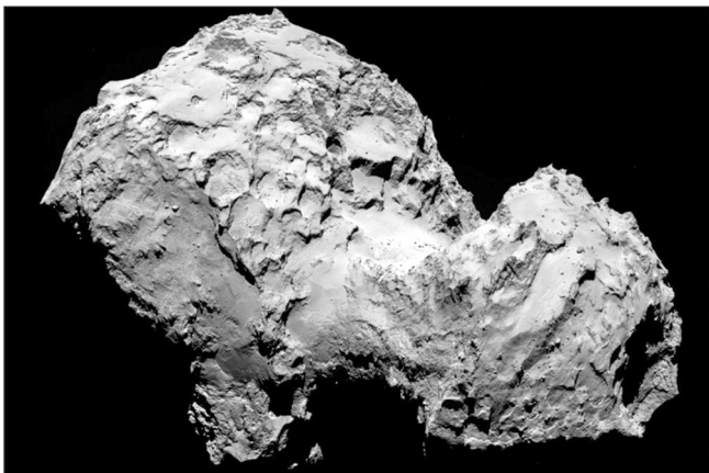
Знімок комети Чурюмова—Герасименко, виконаний КА "Розетта" 03.08.2014 з відстані 285 км
