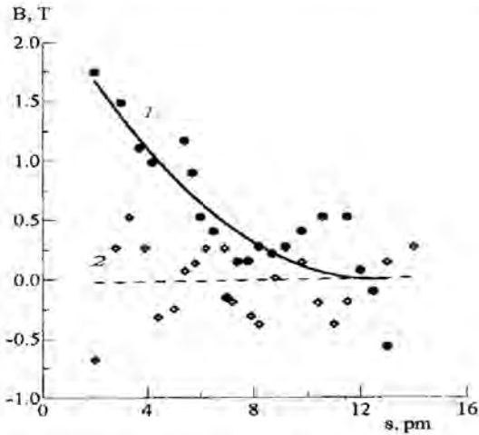
Рис. 1. Сопоставление наблюдаемого расщепления бисекторов профилей I \pm V в линии Fe I 557.61 нм для вспышки 5 ноября 2004 г. (зависимость 1) и нево вспышечной области (зависимость 2). По оси абсцисс дано расстояние s от центра линии в пикометрах, по оси ординат — величина магнитного поля B в тесла (Тл)
