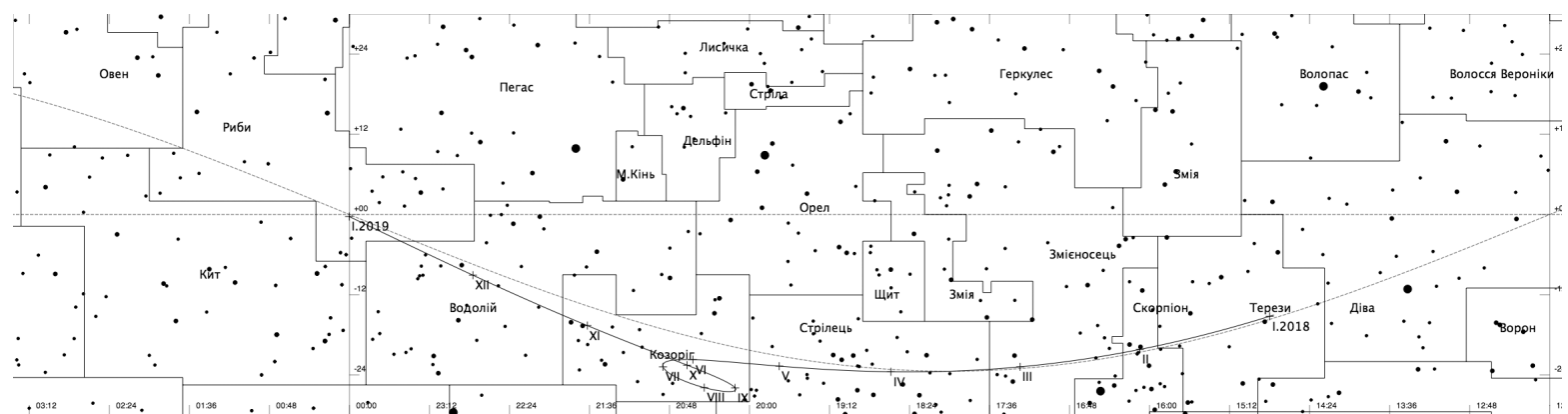
Рис. 7. Видимий шлях Марса
